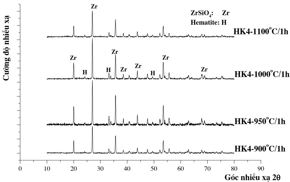
Hình 2: Phổ XRD của mẫu HK4 nung ở các nhiệt độ khác nhau từ 900 ÷ 1100°C
