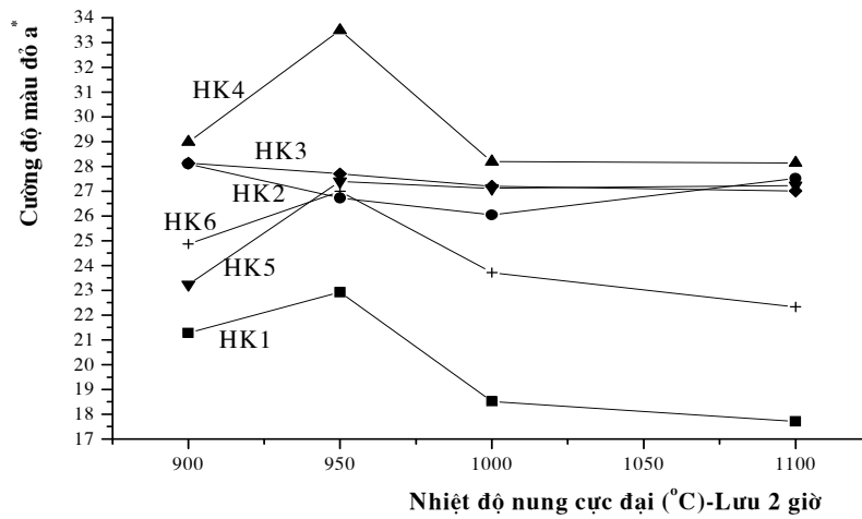
Hình 1: Đồ thị biểu diễn chỉ số a* (màu đỏ) của các mẫu phụ thuộc theo nhiệt độ nung 900 - 1100°C/2h
