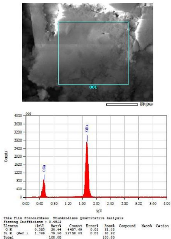
Hình 5: Phổ EDX của vật liệu SN1,5/1
