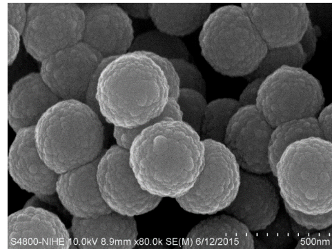
Hình 2: Ảnh SEM của mẫu SN1,5/1 ở góc chụp khác
