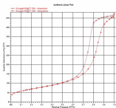
Hình 1a: Đường đẳng nhiệt hấp phụ và khử hấp phụ N 2 của mẫu Co/Silicagel
