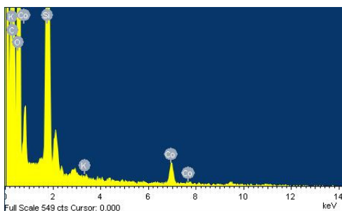
Hình 3c: Phổ EDX của mẫu Co/MCM-41
