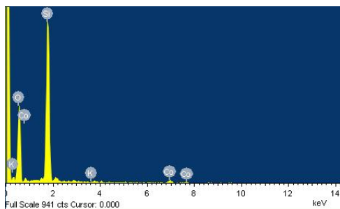
Hình 3a: Phổ EDX của mẫu Co/Silicagel
