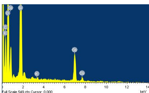
Hình 3b: Phổ EDX của mẫu Co/Silicalit
