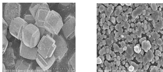
Hình 2b: Ảnh SEM của mẫu Co/Silicalit
