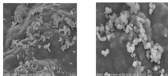
Hình 2c: Ảnh SEM của mẫu Co/MCM-41
