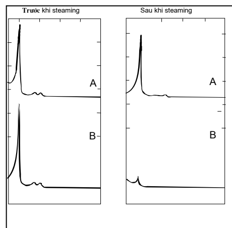
Hình 1: Phổ XRD của các mẫu trước và sau steaming A-mẫu H-Al-MSU; B-mẫu H-Al-MCM41
