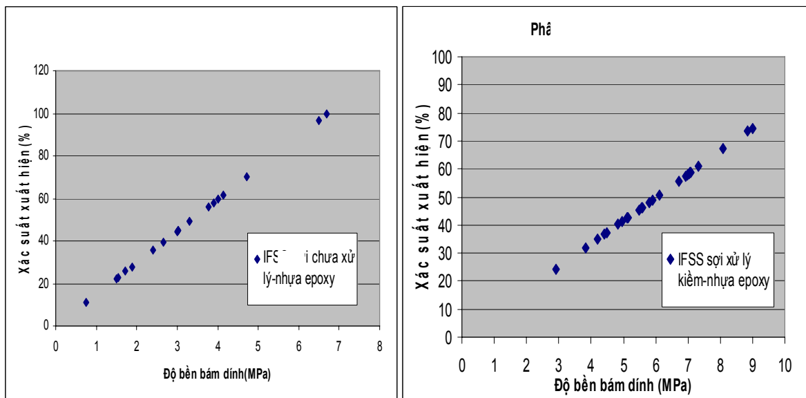
Hình 1: Phân bố độ bền bám dính sợi-nhựa của sợi dứa dại trước và sau khi xử lý kiềm
