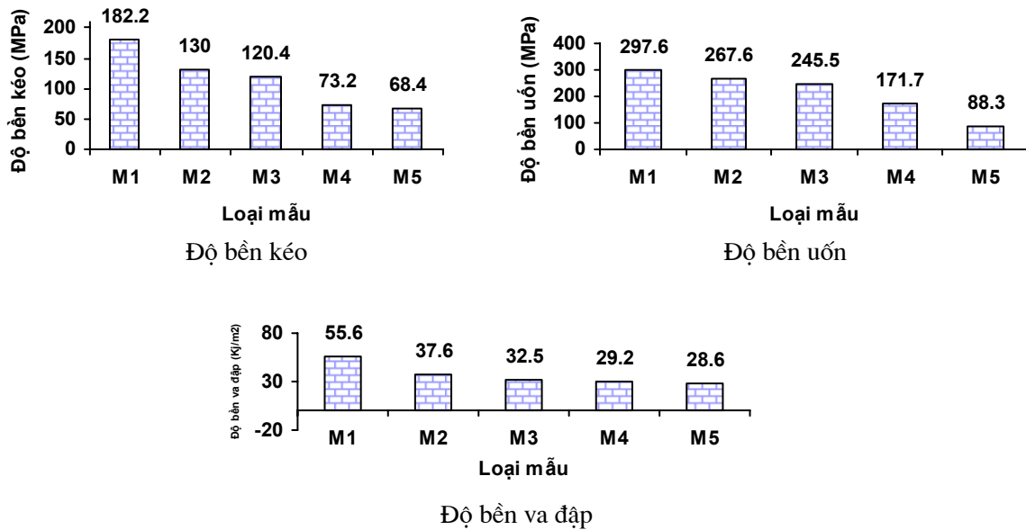
Hình 6: Ảnh hưởng của hàm lượng mat đũa đại/thủy tinh đến tính chất cơ học của vật liệu PC
