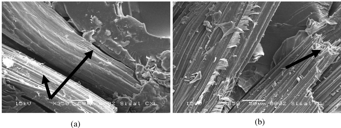
Hình 3: Ảnh SEM chụp bề mặt phá hủy composit sợi chưa xử lý (a) và xử lý kiềm (b)
