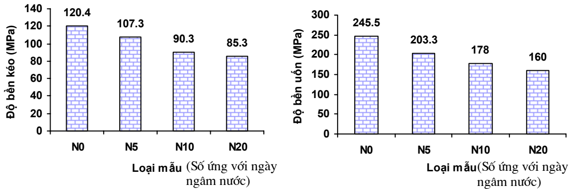
Hình 7: Ảnh hưởng của thời gian ngâm nước đến độ bền kéo và độ bền uốn của vật liệu PC (No - mẫu không ngâm nước)
