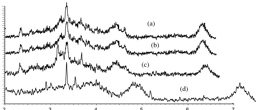
Hình 1: Phổ XRD xúc tác \gamma\text{-Al}_2\text{O}_3 chưa hoạt hóa và đã hoạt hóa \text{Na}_2\text{CO}_3 nung ở 300^\circ\text{C} và 500^\circ\text{C}
