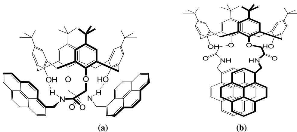
Hình 2: Cấu trúc của dipyrenyl calix[4]aren trong các dung môi khác nhau (a) trong \text{CH}_3\text{CN} ; (b) trong hỗn hợp \text{H}_2\text{O}/\text{CH}_3\text{CN} (4:1, v/v)
