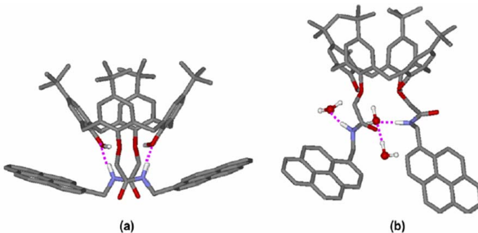
Hình 3: Cấu trúc của dipyrrenyl calix[4]aren mô phỏng theo lý thuyết hàm mật độ (a) dipyrrenyl calix[4]aren trong chân không; (b) dipyrrenyl calix[4]aren khi có mặt 3 phân tử nước
