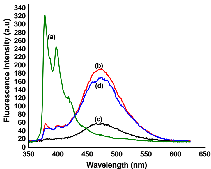
Hình 1: Phổ huỳnh quang của 1 và phức 1 .Fe(III) (nồng độ của 1 là 2,5 \mu\text{M} và của \text{Fe}^{3+} là 75 \mu\text{M} )
