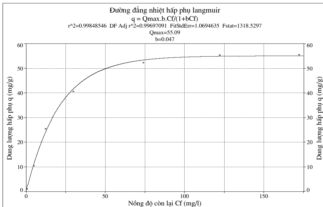
Hình 3: Đường đẳng nhiệt hấp phụ As(III) của \text{LaFeO}_3 kích thước nanomet
