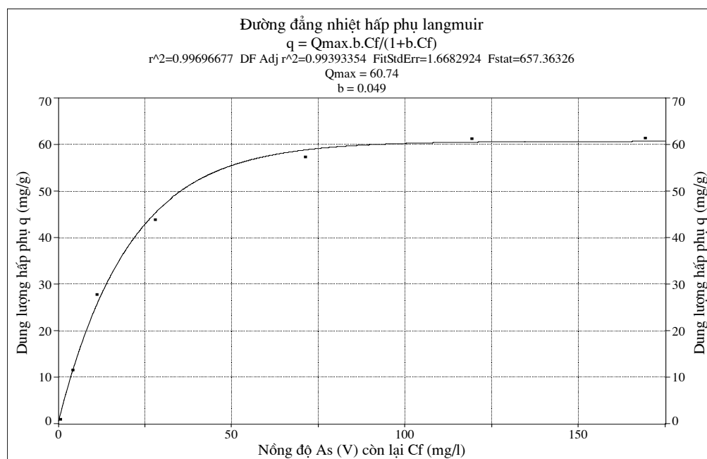
Hình 4: Đường đẳng nhiệt hấp phụ As(V) của \text{LaFeO}_3 kích thước nanomet
