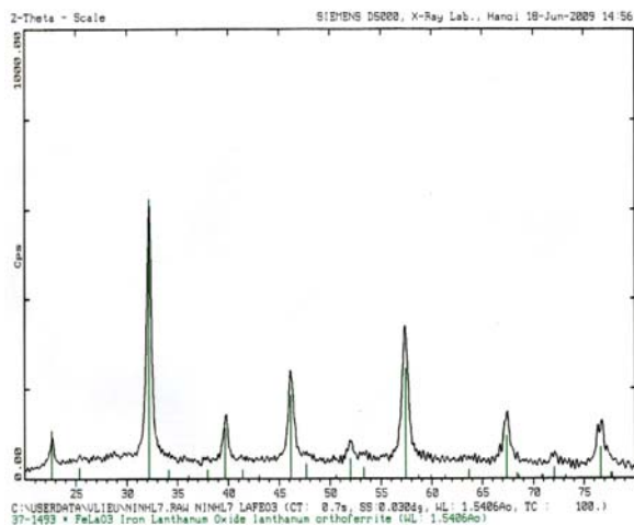
Hình 1: Phổ nhiễu xạ tia X của \text{LaFeO}_3
