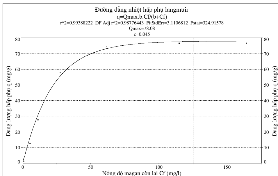
Hình 6: Đường đẳng nhiệt hấp phụ \text{Mn}^{2+} của \text{LaFeO}_3 kích thước nanomet
