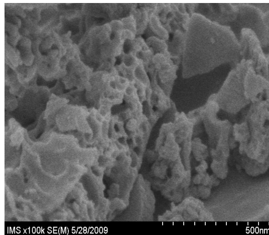
Hình 2: Ảnh SEM của \text{LaFeO}_3
