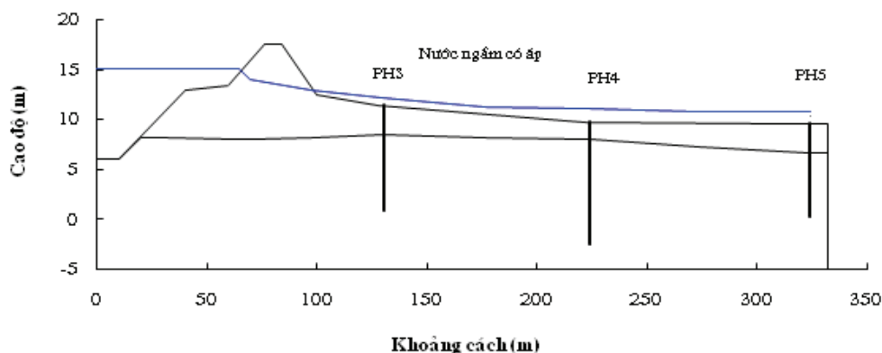
Hình 5. Mức nước áp lực trong đồng khi lũ lên tại K32+960
