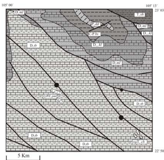
Hình 5. Sơ đồ cấu trúc địa chất vùng quặng Na Sơn
