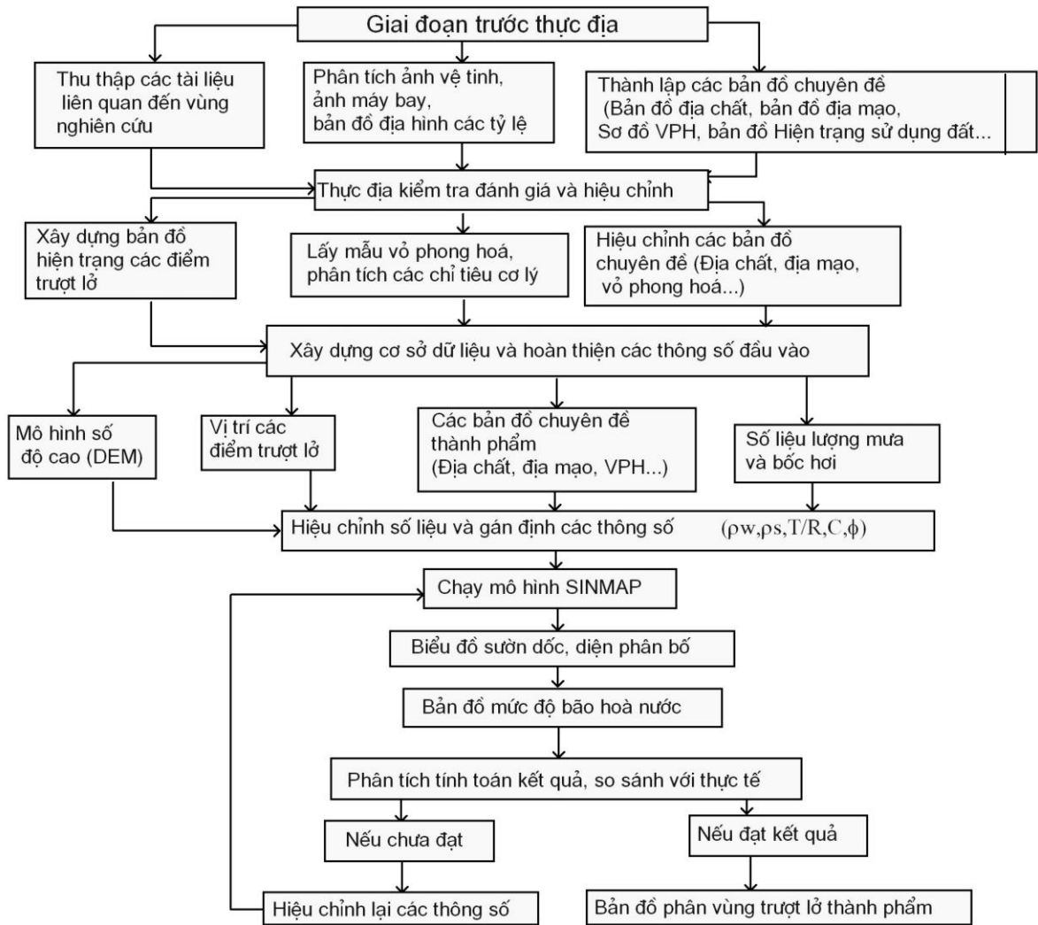
Hình 3. Sơ đồ khối của mô hình SINMAP
