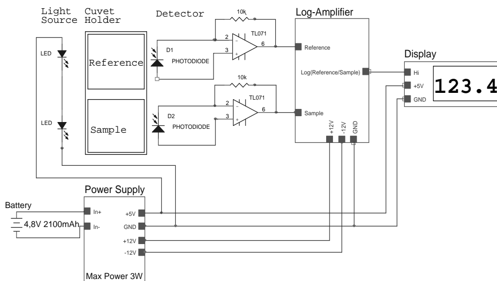
Hình 1: Sơ đồ mạch nguyên tắc hoạt động của máy PN01
