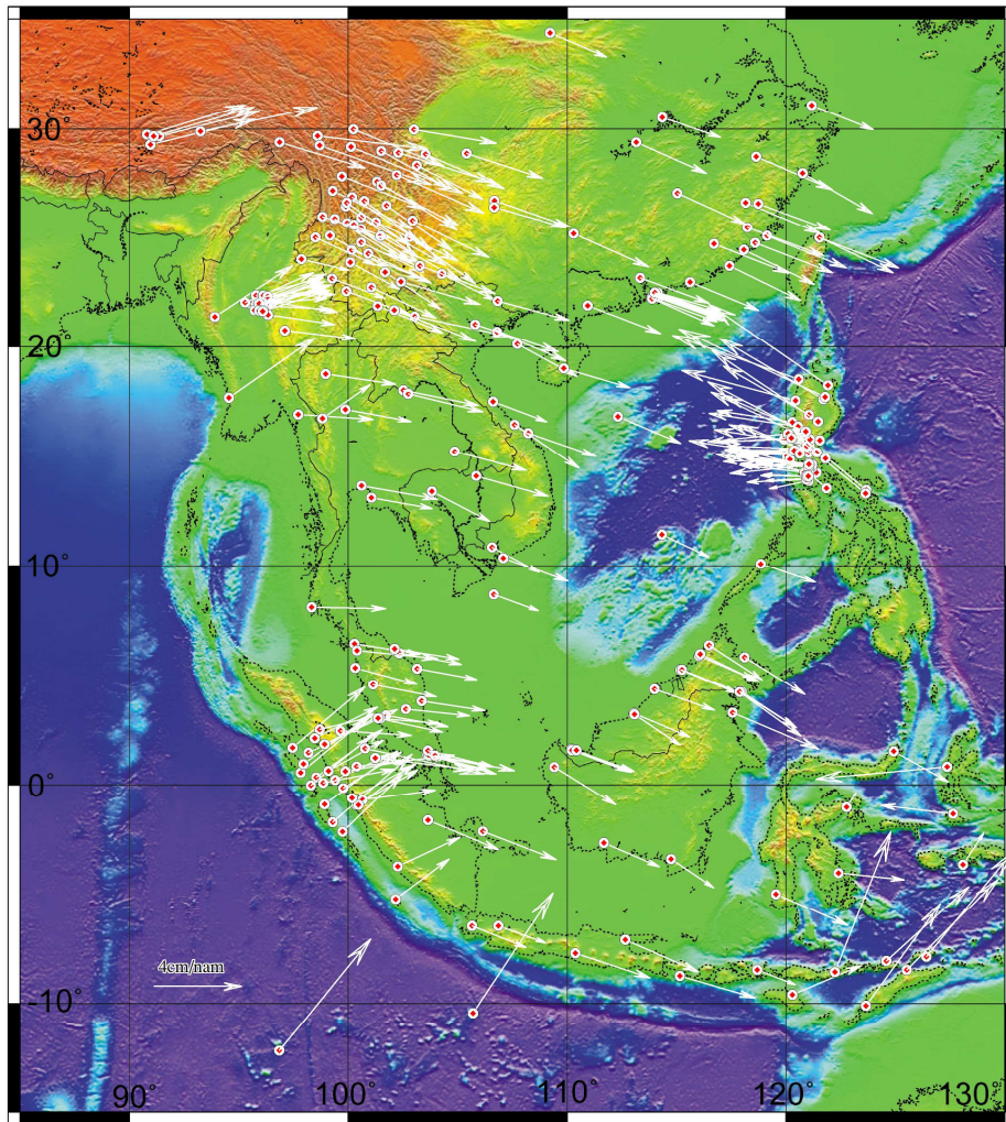
Hình 2: Sơ đồ tổng hợp các vec tơ vận tốc chuyển động kiến tạo hiện đại theo kết quả đo của chương trình GEODYSSSEA, chương trình PCGIAP, chương trình SEAMERGES, chương trình CMONOC, Beavan và nnk., 2004, Bock và nnk., 2003, Chamote-Rooke, 1999, Dawson và nnk., 2004, Gan và nnk., 2007, Galgana và nnk., 2007, Iwakuni và nnk., 2004, Michel và nnk, 2001, Shen và nnk, 2005, Simos và nnk., 2007, Socquet và nnk, 2006, Rangin và nnk., 1999. Zhang và nnk, 2004 và kết quả đo GPS của tập thể tác giả bài báo này
