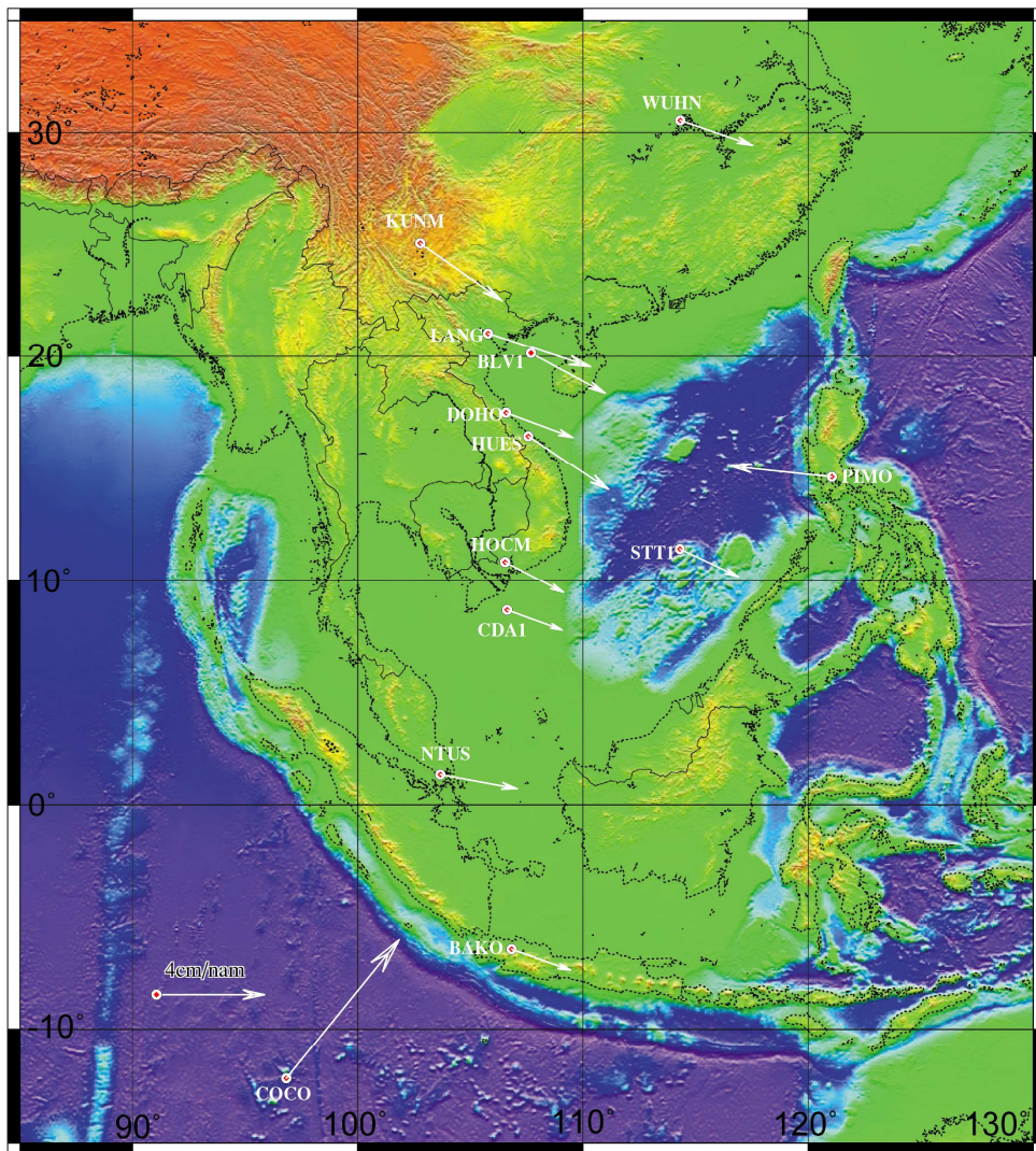
Hình 1: Sơ đồ tốc độ chuyển dịch tuyệt đối trong IGS05 của các trạm GPS trên Biển Đông, theo 3 đợt đo các năm 2007 - 2008 - 2009
