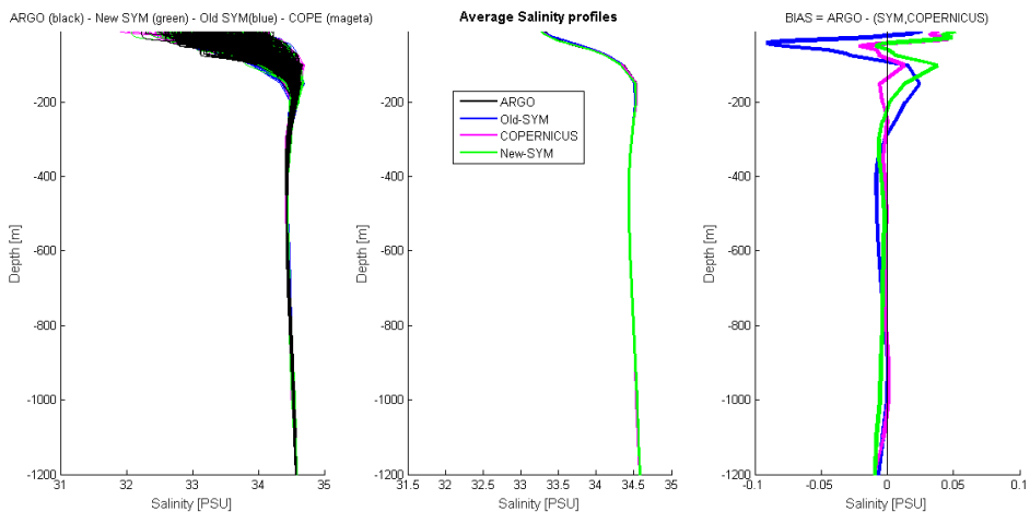
Hình 13. Phân bố thẳng đứng độ muối của mô hình chưa hiệu chỉnh (xanh lam), đã hiệu chỉnh (xanh lục), COPERNICUS (tím) tương ứng với các trạm ARG0 (đen) trong năm 2014. Profile tổng cộng độ muối (trái), trung bình (giữa) và độ lệch trực tiếp với ARG0 (phải) của các bộ dữ liệu với thực đo
