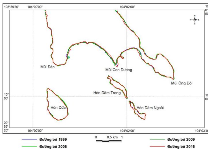
Hình 4. Các thể hệ đường bờ giai đoạn 1999–2016
