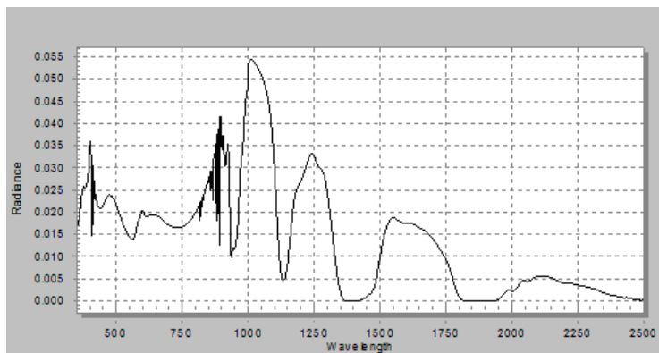
Hình 5. Đặc trưng quang phổ san hô, cỏ biển phát triển tốt khu vực đảo Nam Yết
